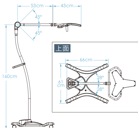
●キャスタースタンド型寸法図
