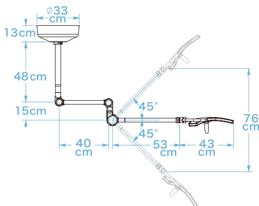
●天井吊下げ型寸法図
